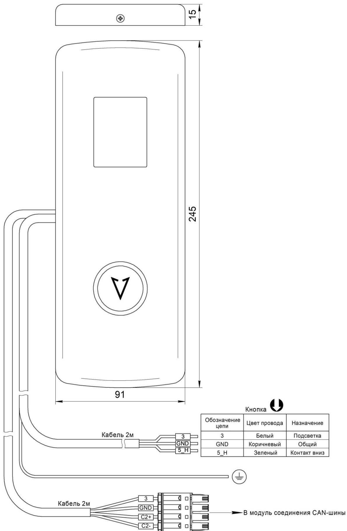
Рис.1 Внешний вид, габаритные и установочные размеры Вызывного поста ЦИРКОН НШЕК.468381.035-01
